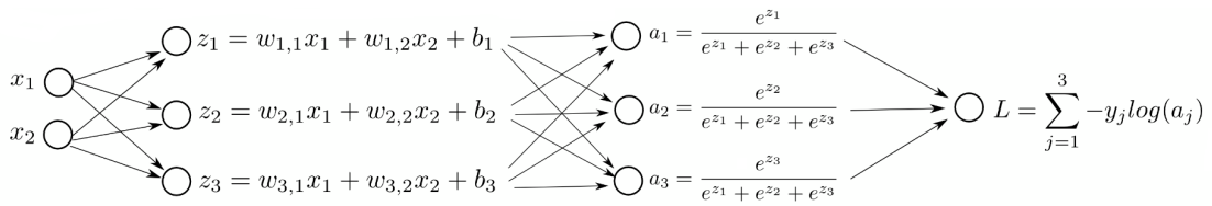
Figura 4.2: Flusso della regressione softmax con due ingressi e tre classi: dai logiti z_i = w_{i,1}x_1 + w_{i,2}x_2 + b_i alle probabilità a_i = \frac{e^{z_i}}{\sum_{k=1}^3 e^{z_k}} , fino alla loss a entropia incrociata L = \sum_{j=1}^3 -y_j \log(a_j) .
